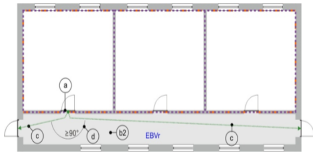
Figuur 12: Twee vluchtroutes linker vleugel
