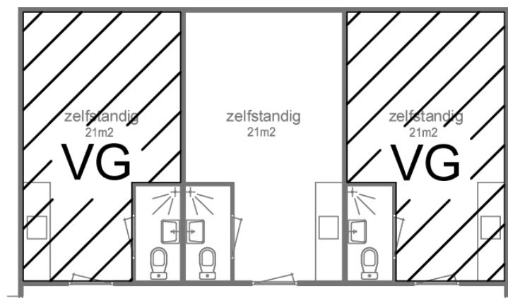
Figuur 13: Positie van verblijfsgebieden (VG) in voorbeeldplattegrond
