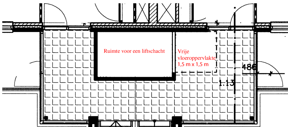
Figuur 17: Vrije vloeroppervlakte voor lifttoegang
