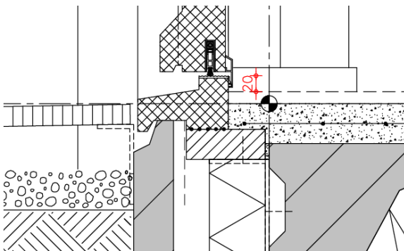
Figuur 18: Voorbeeld van een 20 mm - detail
