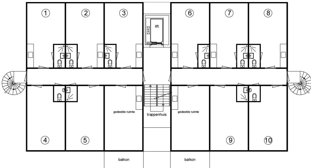
Figuur 4: Voorbeeld plattegrond gebouwindeling studentenhuisvesting
